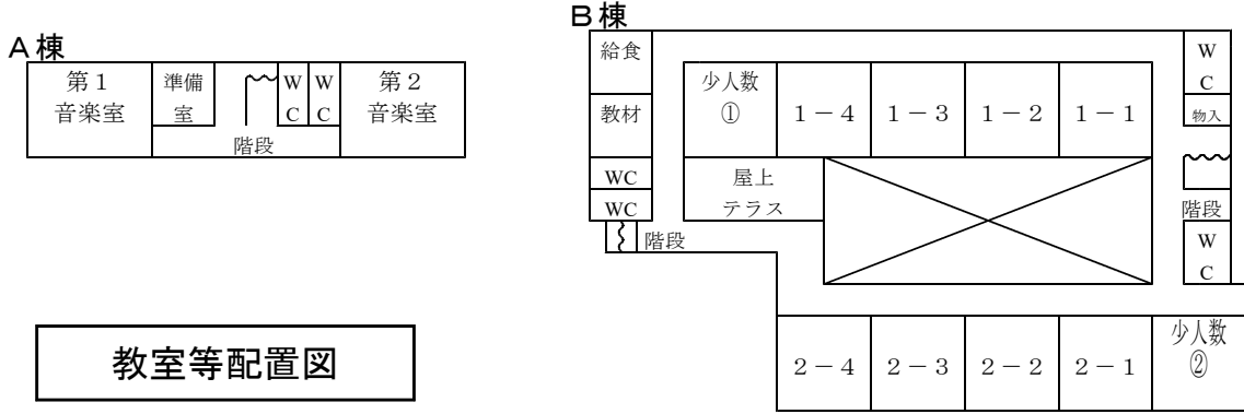
校舎配置図
